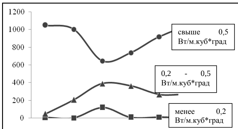
Рис. 12. Динамика количества зданий с разными показателями удельной поставки в течение отопительного периода 2013/2014 гг.
