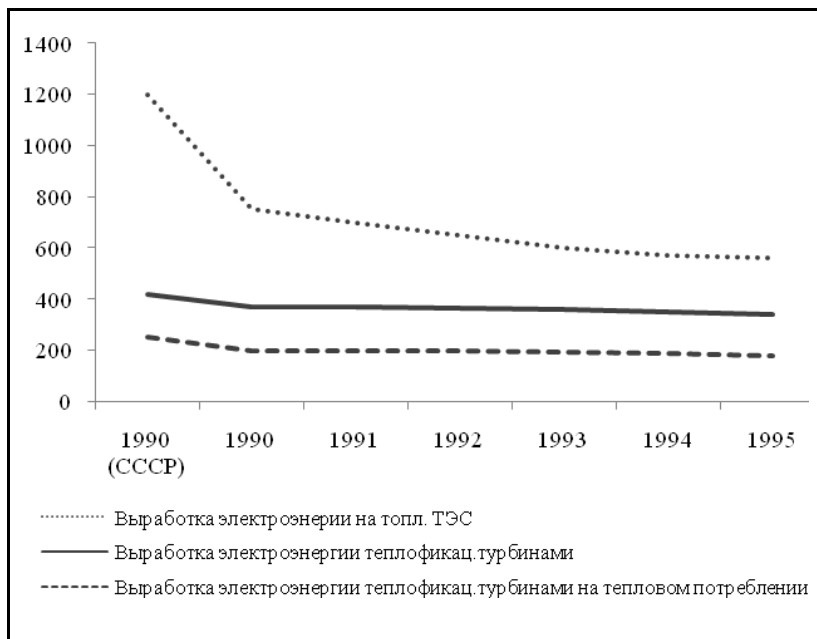
Рис. 4. Динамика падения выработки электроэнергии на ТЭС общего пользования и на ТЭЦ на рубеже 1990-1995 гг.
