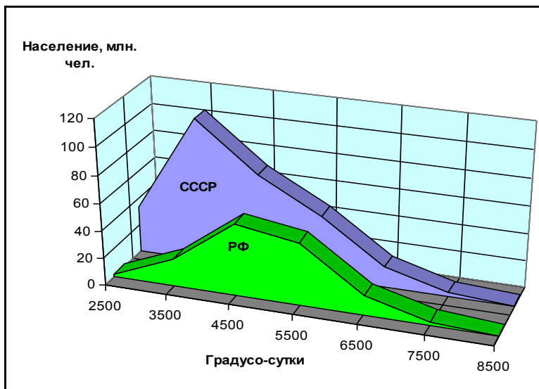
Рис. 2. Распределение населения СССР и РФ по градусо-суткам отопительного периода
