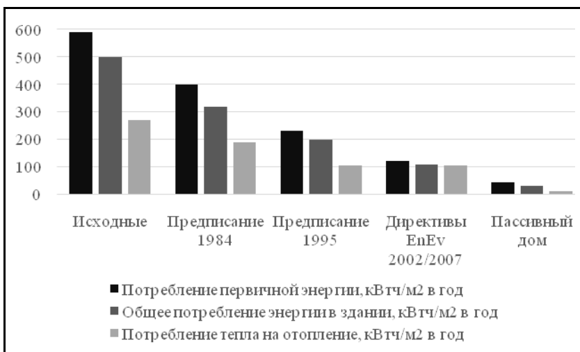
Рис. 17. Ужесточение требований к потреблению зданиями энергии
