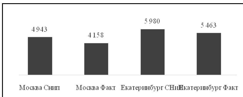
Рис. 6б. Сокращение градусо-суток отопительного периода
