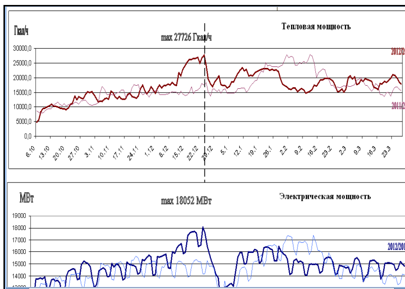
Рис. 13. Динамика потребления тепловой и электрической мощности в Московском мегаполисе
