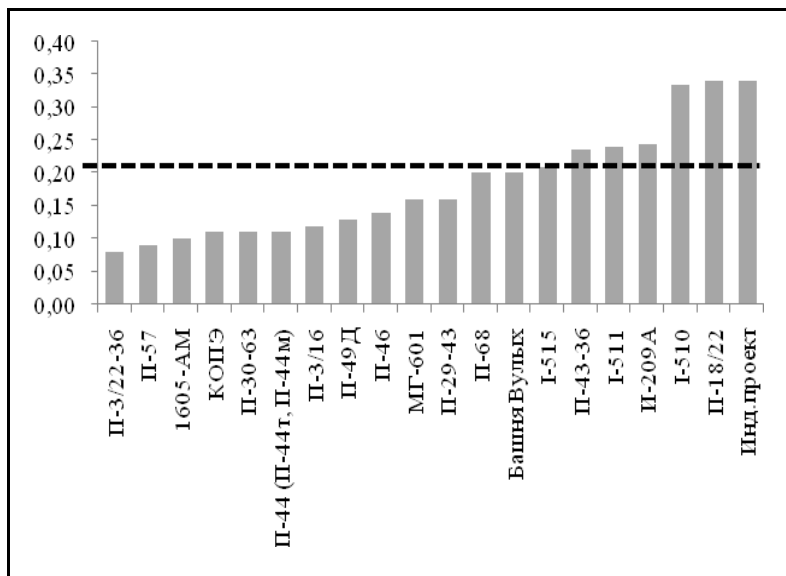
Рис.11. Показатели удельного потребления тепла на отопление зданий разных серий
