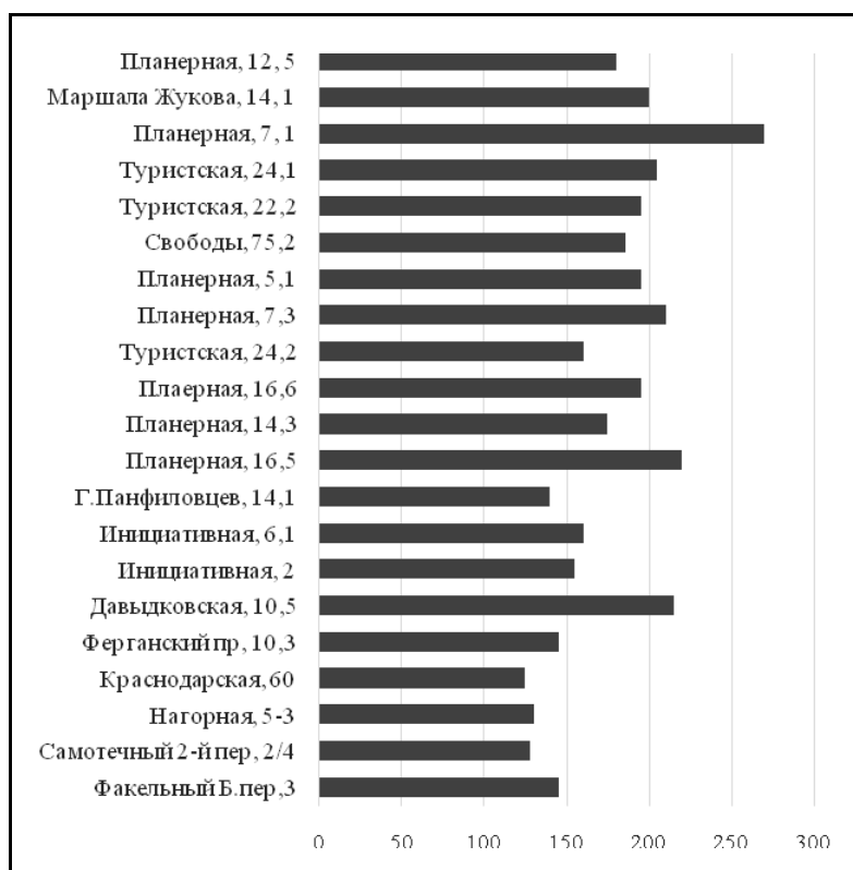
Рис. 10. Удельное потребление тепловой энергии на отопления в зданиях после капитальных ремонтов (г. Москва)
