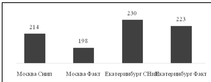
Рис. 6а. Изменение суток отопительного периода для Москвы и Екатеринбурга
