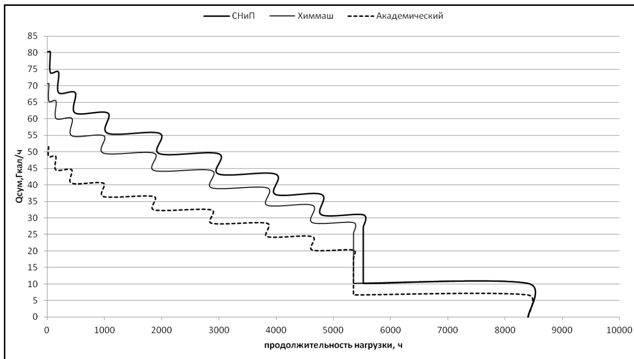
Рис. 8. Изменение графика тепловой нагрузки зданий мегаполиса (г.Екатеринбург) за счет суммарных климатических и строительных факторов
