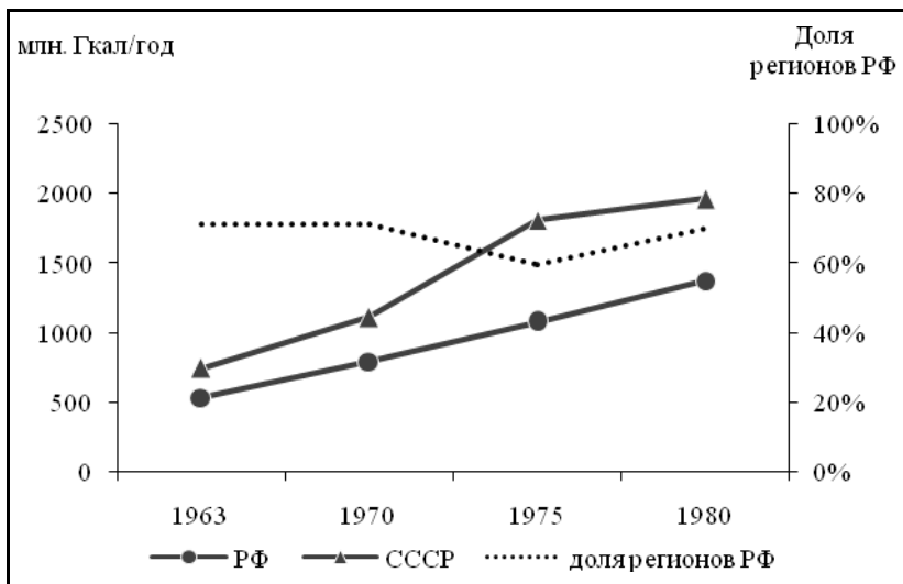
Рис. 1. Суммарное теплотребление регионами РФ и СССР в целом
